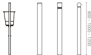
Typy sloupků / Post
