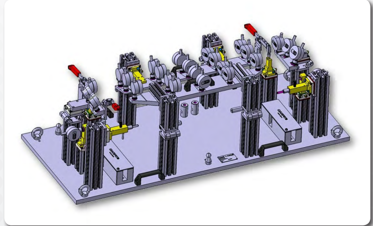
Měřicí, upínací přípravky a cubingy
