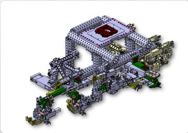
Montážní a manipulační efekторы
